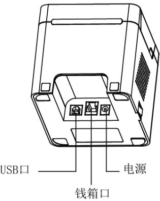
接口说明
